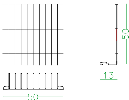
nr. 2 pz. Lateralì lunghi 50 x H. 50 cm
