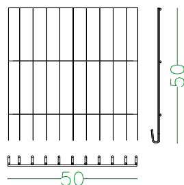
nr. 2 pz. Lateralì corti 50 x H. 50 cm
