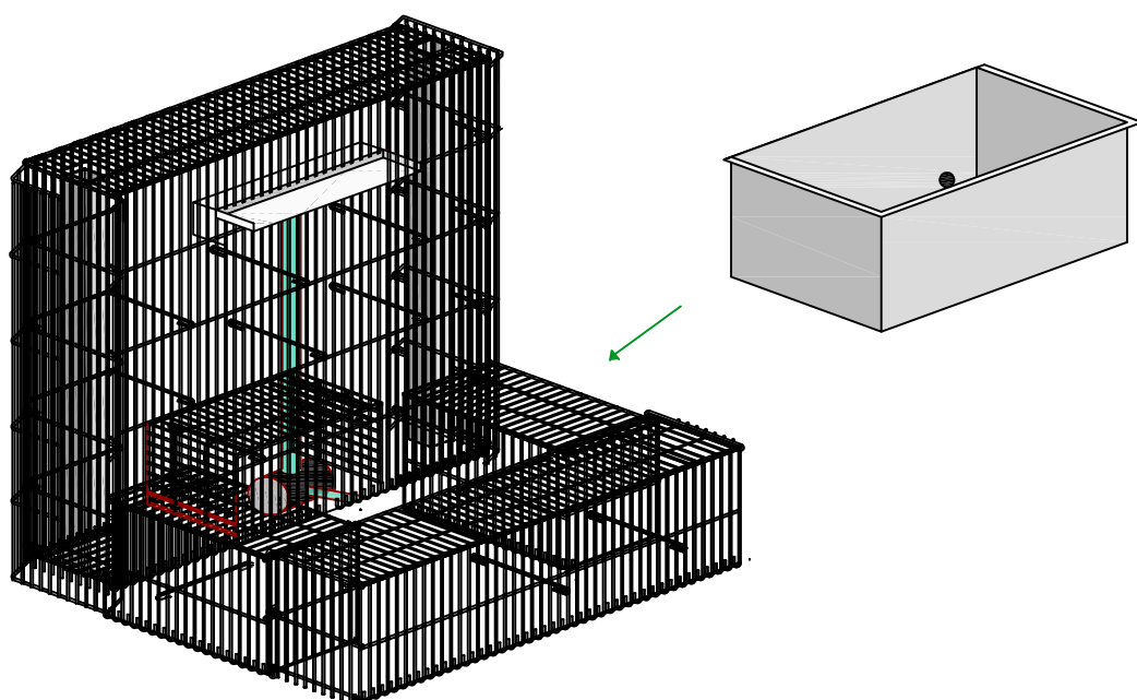
STEP 8 posizionamento della vasca e collegamento alla pompa
